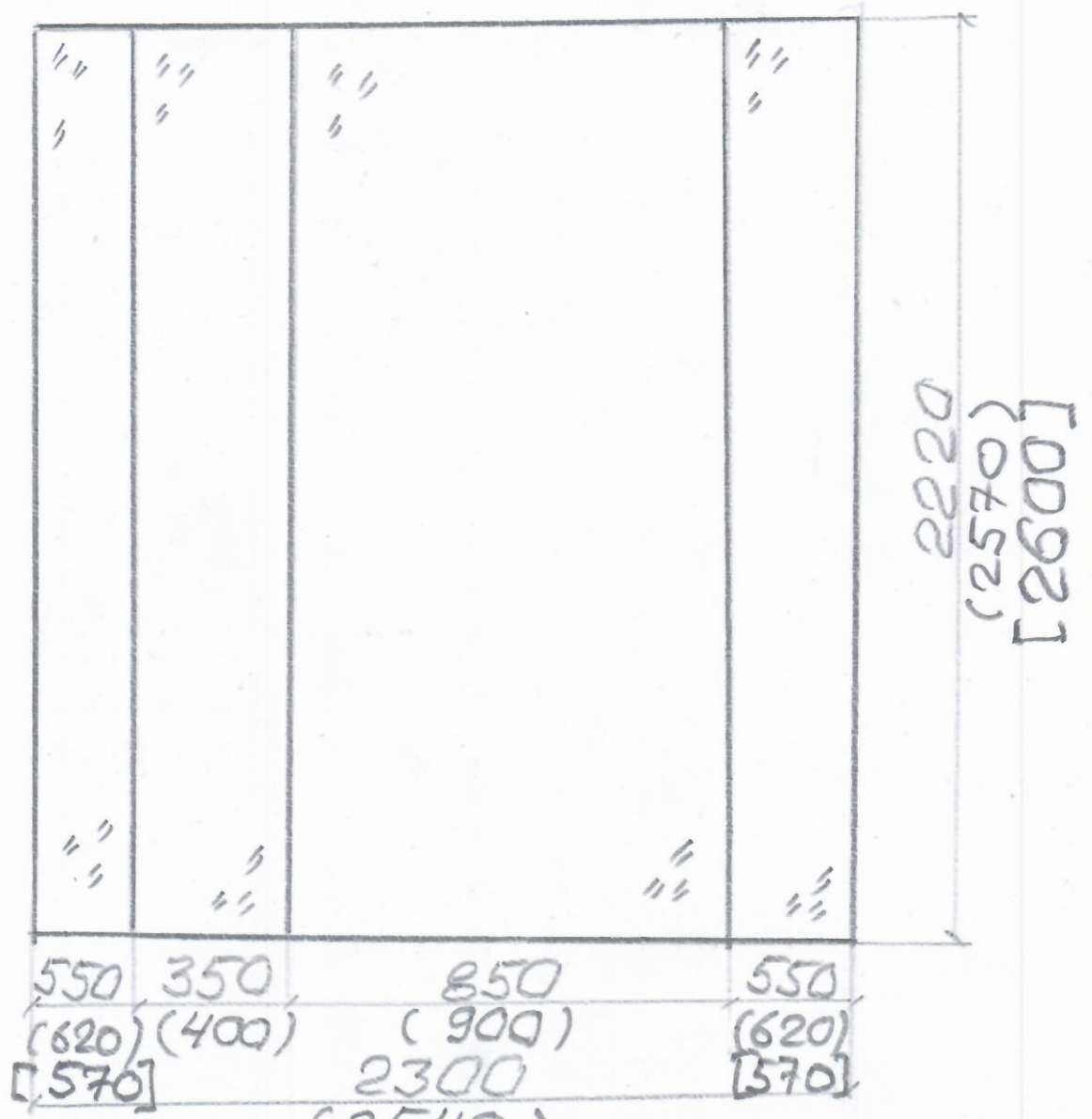
Рисунок 2 Перегородка с двухстворчатой дверью со стеклопакетом
