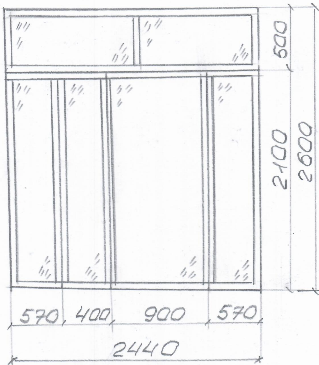
Рисунок 5 Терзгородіса с двухстворчатой дверью со стеклопакетом
