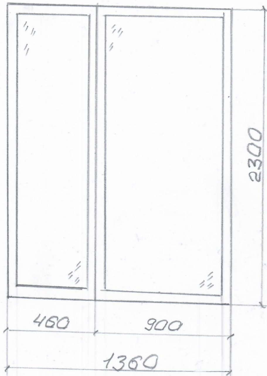
Рисунок 1 Дверь двухстворчатая УК 1 - ауд - 1/234 1-шт
