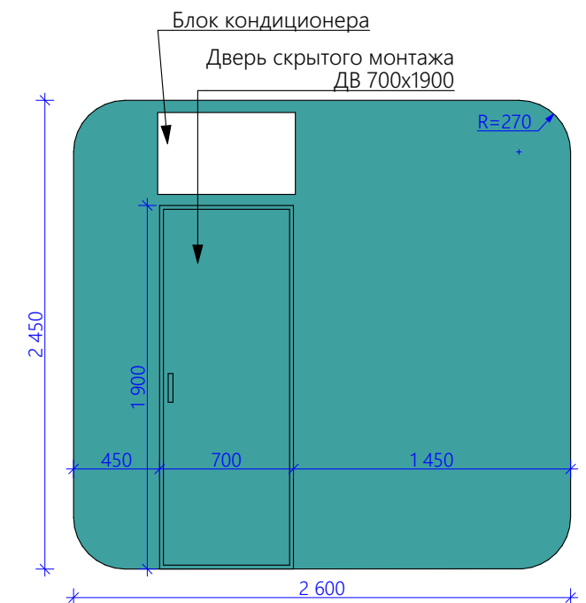
Вид сзади
