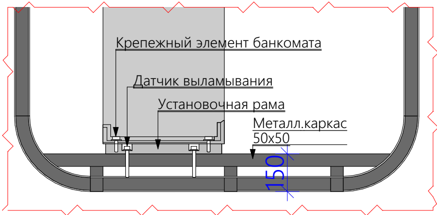
Узел А
