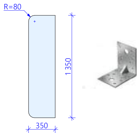
Крепеж перегородки(каленое стекло) на уголок
