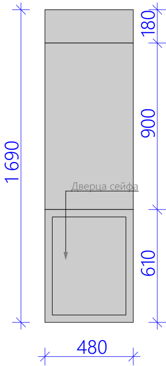
Вид сзади
