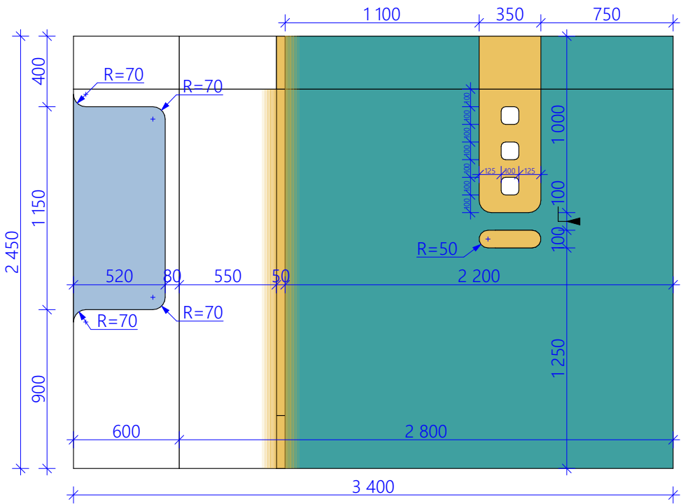
Боковой вид 02 (второй вариант)
