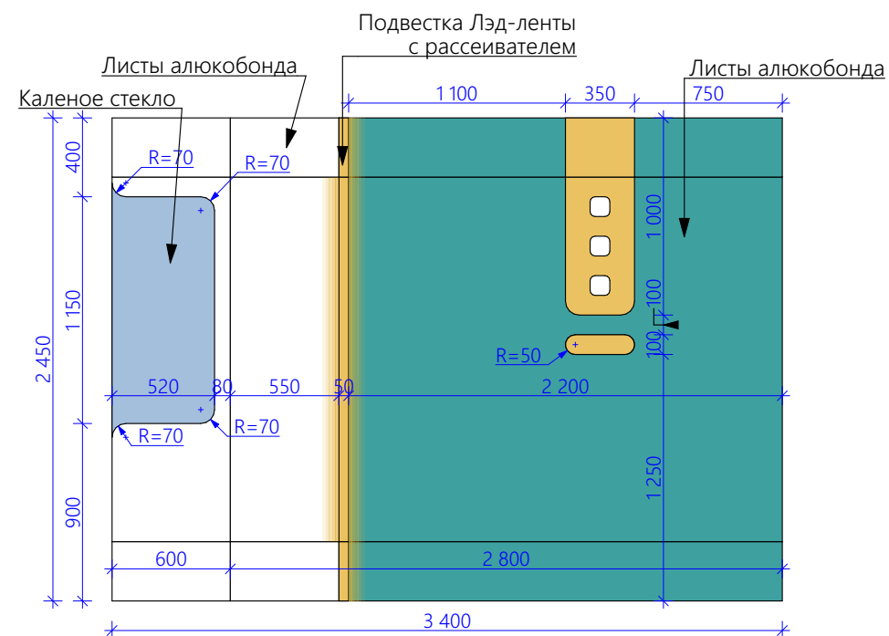
Боковой вид 02
