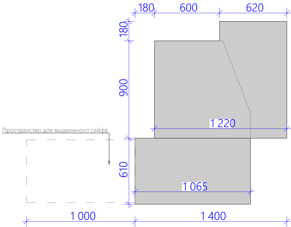
Боковой вид
