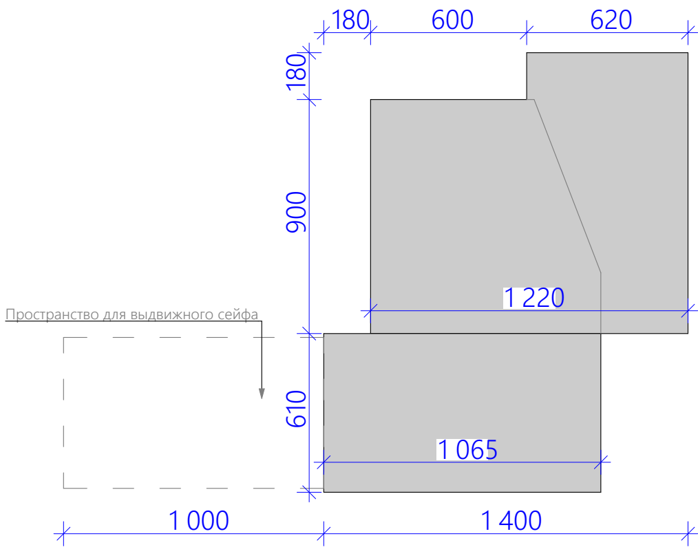
Боковой вид
