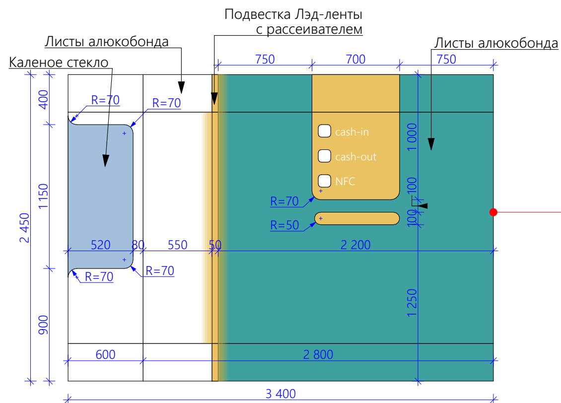
Бокковой вид 02 (первый вариант)
